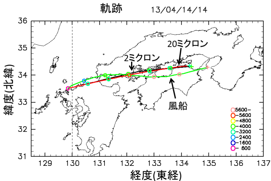
図8 放射性微粒子の初期高度が3000 mであること以外は図6と同じ
