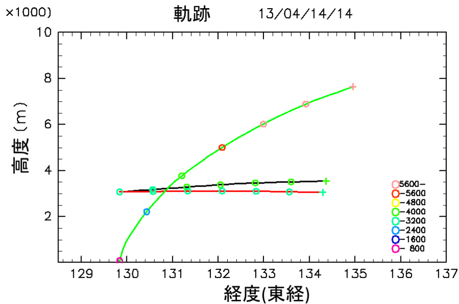
図9 放射性微粒子の初期高度が3000 mであること以外は図7と同じ
